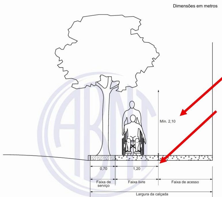
Figura 90 – Faixas de uso da calçada – Corte
