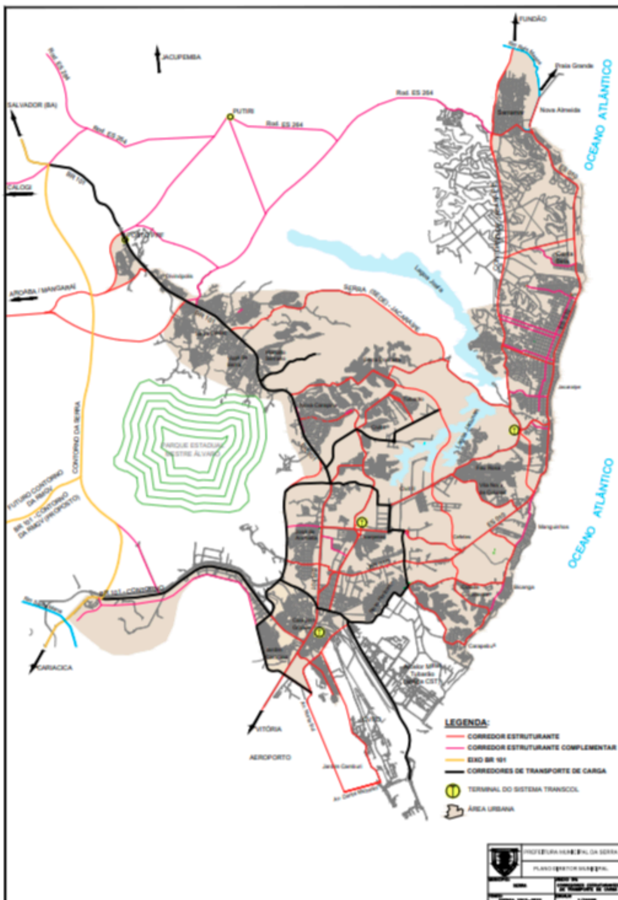
Figura 12: Corredores de transporte de carga
